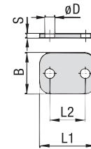
STAUFF Größe 1A bis 8
